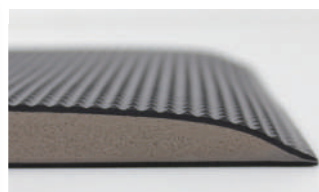
耐摩耗・発泡・防水層の三層構造で 水・油の吸収を防ぎ キャスターが通過しやすい傾斜構造。
